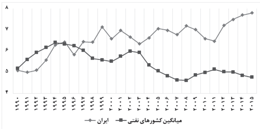
نمودار ۱۴-۷. مقایسه شدت انرژی ایران و میانگین کشورهای نفتی در دوره ۱۹۹۰ تا ۲۰۱۵
