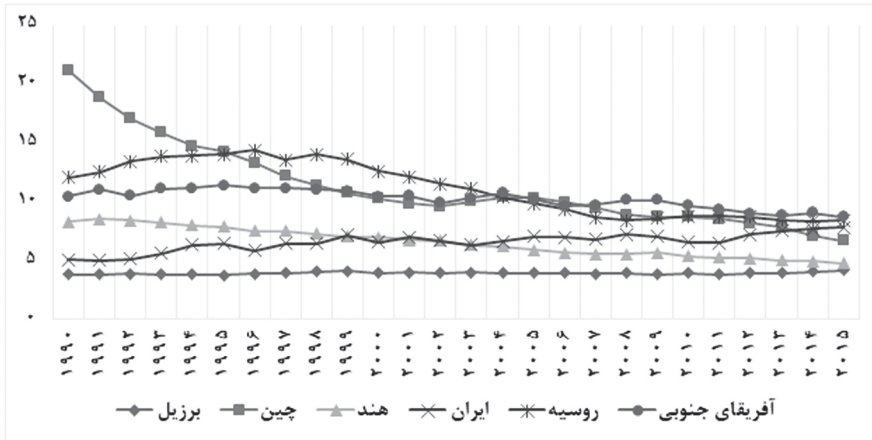
نمودار ۱۴-۶. شاخص شدت انرژی ایران در مقایسه با اقتصادهای نوظهور
