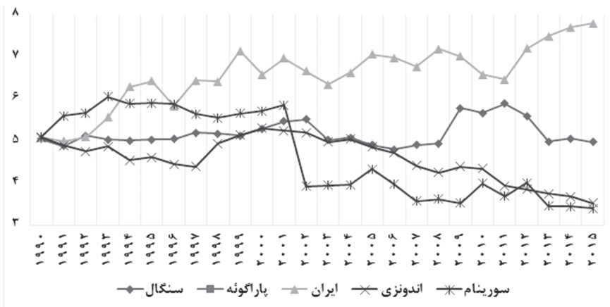
نمودار ۱۴-۴. مقایسه شدت انرژی در ایران با کشورهای نزدیک به آن
