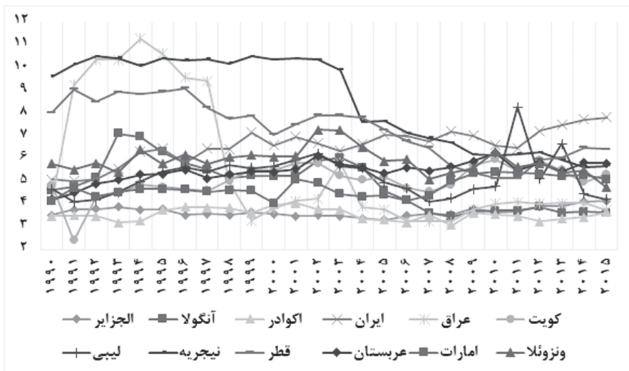
نمودار ۱۴-۸. مقایسه شدت انرژی ایران و کشورهای نفتی در دوره ۱۹۹۰ تا ۲۰۱۵
