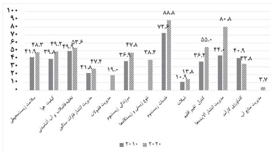
نمودار ۱۲-۳. مقایسه زیرشاخص‌های عملکرد زیست‌محیطی ایران در دو سال ۲۰۲۰ و ۲۰۱۰
