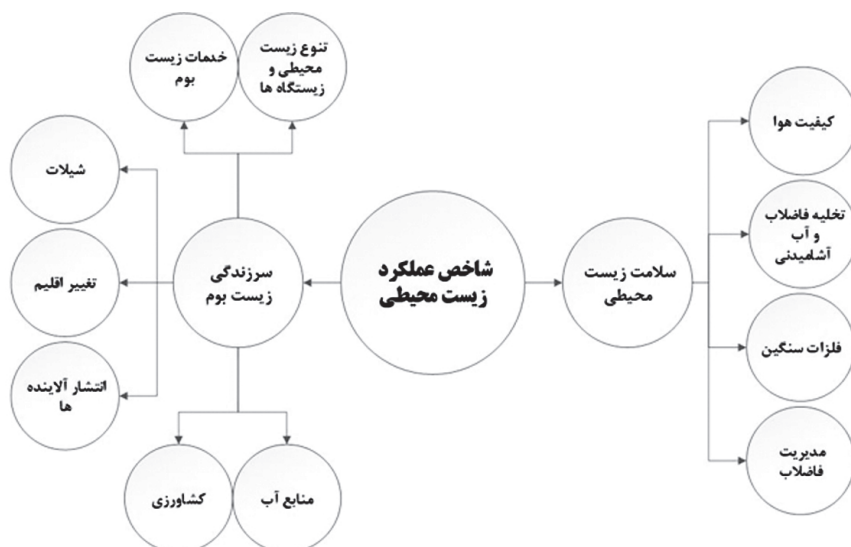
نمودار ۱۲-۱. اجزای شاخص عملکرد زیست محیطی
