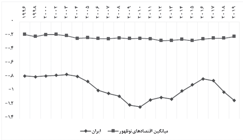
نمودار ۲-۷. شاخص حکمرانی ایران در مقایسه با میانگین اقتصادهای نوظهور
